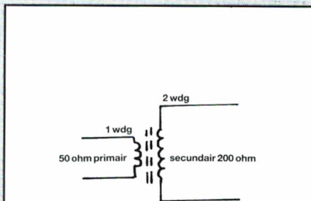
FIG. 15. Transformeren van impedanties. De overzetverhouding is het kwadraat van de wikkerverhouding
